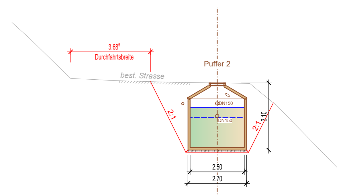
Schnitt B-B 1:100
